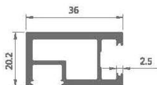
HY-077 后立柱
