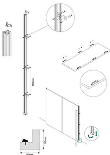
立柱/立柱底座/立柱固定件/背板卡扣
