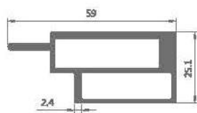
HY-069 前横梁
