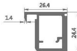
HY-136 25边框
