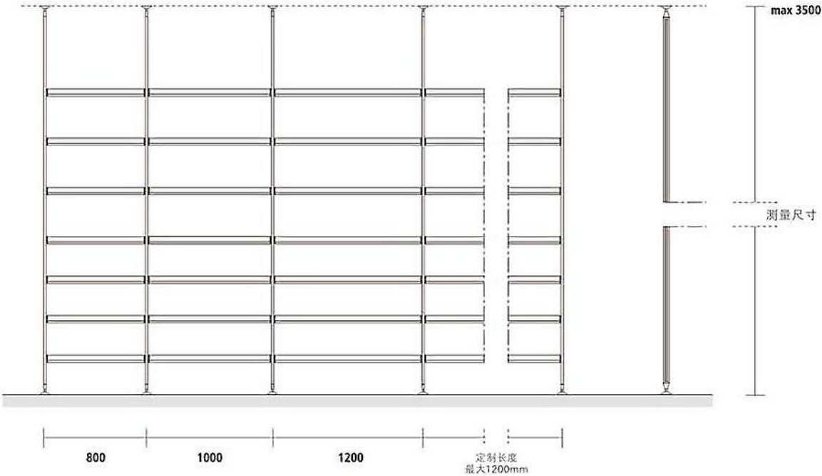
K1书柜立面及剖面示意图
