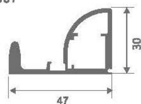
HY-607
