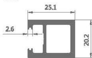
HY-070 35中横
