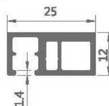
HY-130 25层板边
