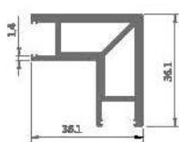
HY-080 转角
