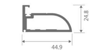
HY-110
