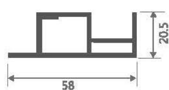
HY-4061
