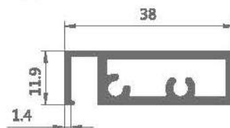
HY-004 36层板边
