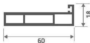
HY-5124
