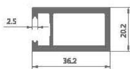
HY-065 前立柱
