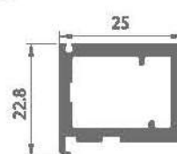
HY-118 25全隐框
